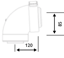
F8 - 87° bend
